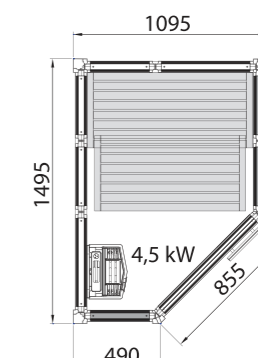
IMPRESSION-SAUNAKABINE I1115/C
