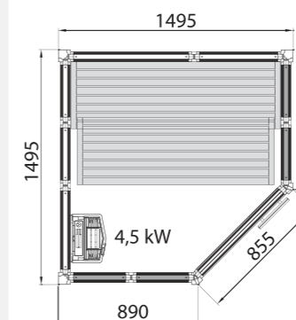
IMPRESSION-SAUNAKABINE I1515/C
