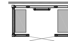
PANACEA 1709 Abmessungen: 1725 x 925 x 2090 mm
