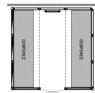
PANACEA 2525 2B Abmessungen: 2525 x 2525 x 2090 mm
