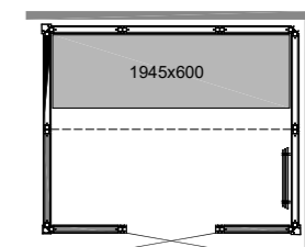
PANACEA 2117 1B Abmessungen: 2125 x 1725 x 2090 mm
