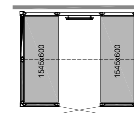
PANACEA 2117 2B Abmessungen: 2125 x 1725 x 2090 mm
