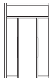
Blockrahmen BR 2 Seitenteile GEHO
